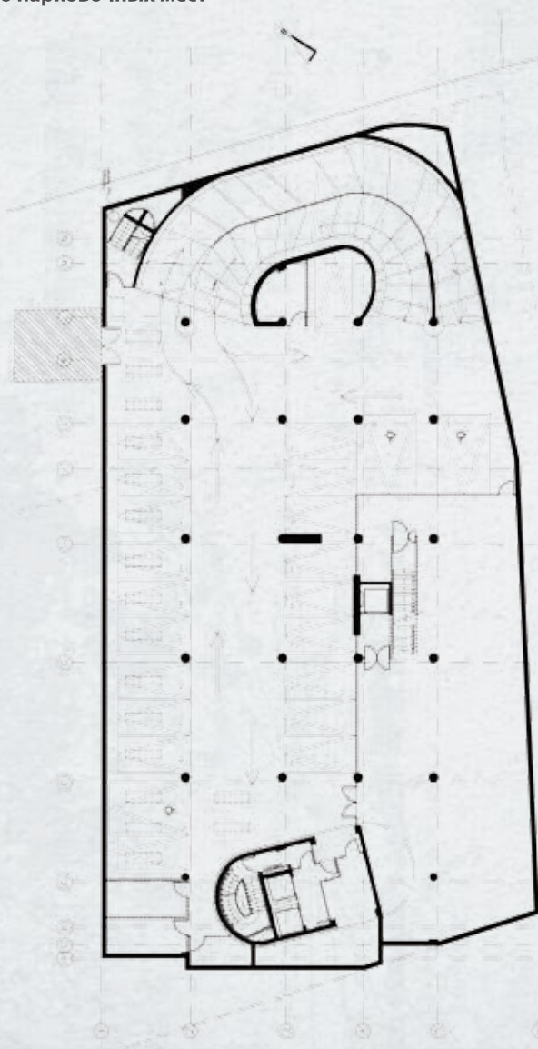
Basement A / Подвальное помещение A
